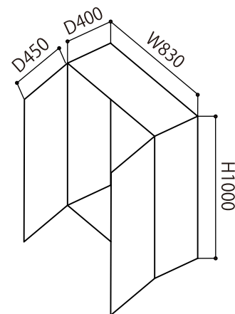
内寸法
